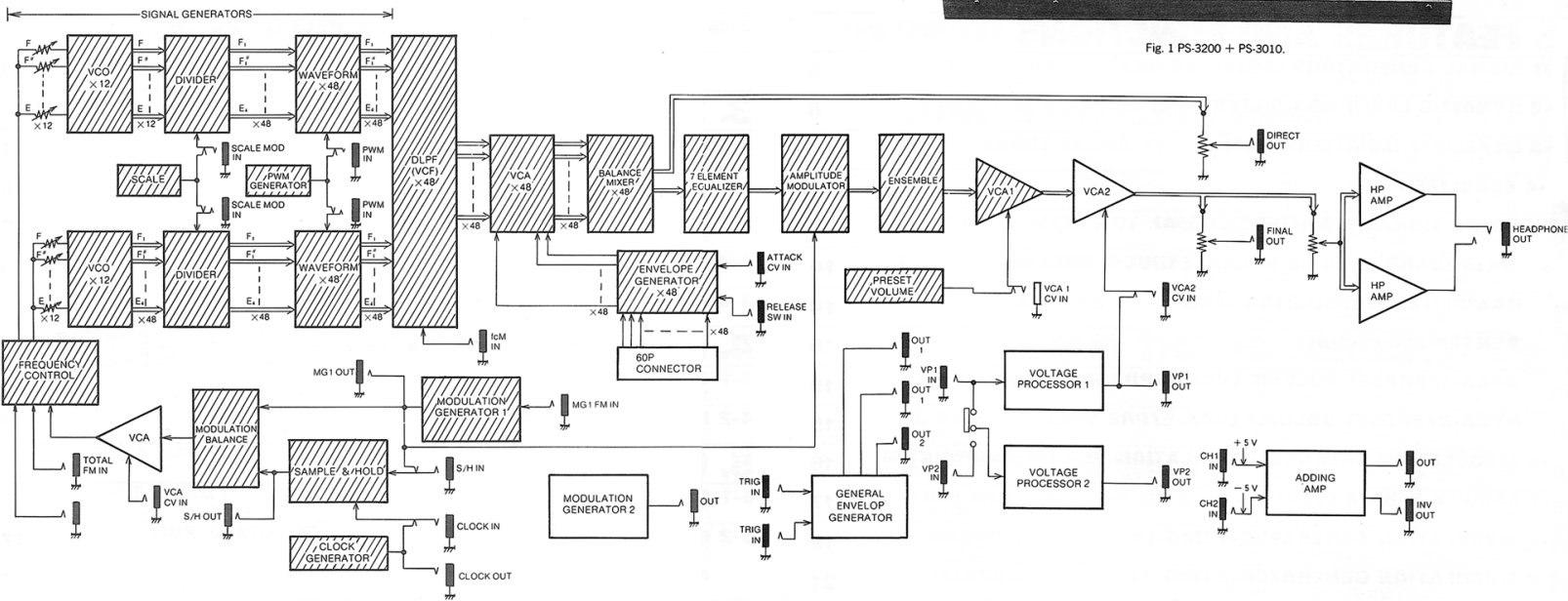
Fig. 2 Block Diagram. ブロックダイアグラム
