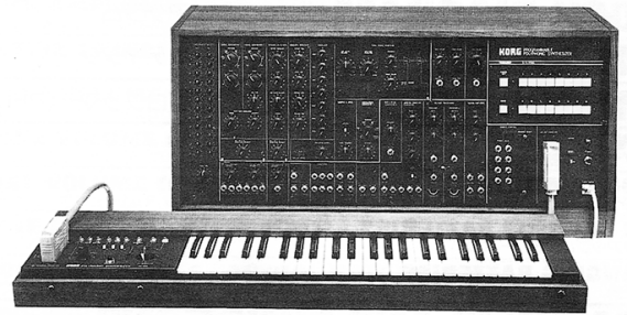
Fig. 1 PS-3200 + PS-3010.
