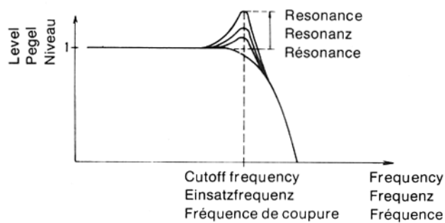
VCF-Frequenzempfindlichkeit
