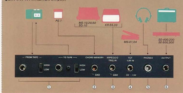
●コルグポリシックスの入出力部分との接続例
