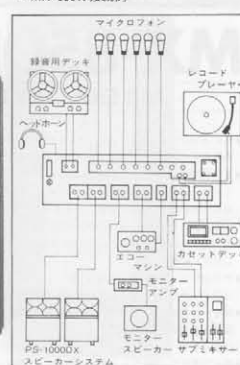
●MX-850の接続例
